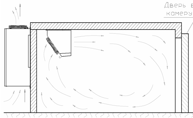
Рис. 3 Пример размещения холодильных машин
