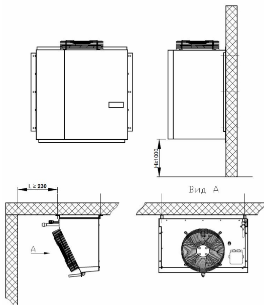
Рис. 4 Монтаж
